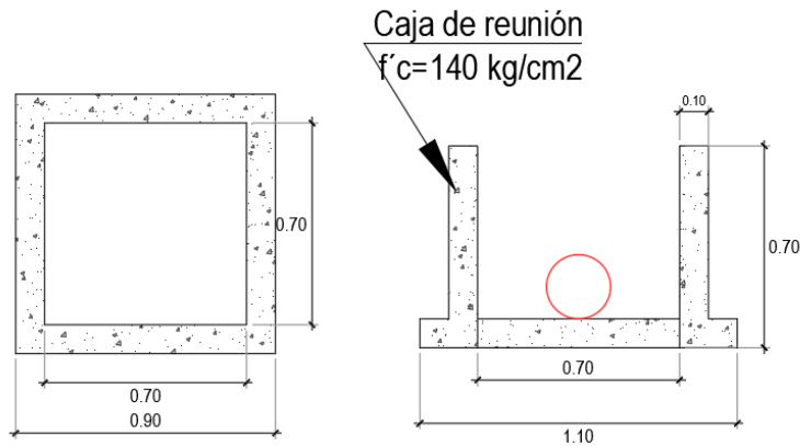
CAJA DE REUNION - CAPTACION DE TUBERIA Escala 1:20
